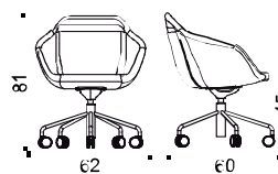
Art 44H/44M: 5-vingat stålstativ med hjul och vipp, roterbart, fast höjd / 5-star steel base with castors and tilt, rotatable, fixed height.
