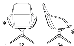
Art 32H/32M: 4-vingat aluminiumstativ glidfötterl och vipp, roterbart, fast höjd / 4-star aluminum base with glides, swivel and tilt, fixed height.
