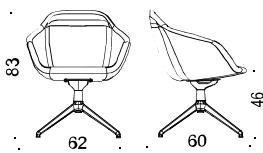
Art 32H/32M: 4-vingat aluminiumstativ glidfötterl och vipp, roterbart, fast höjd / 4-star aluminum base with glides, swivel and tilt, fixed height.
